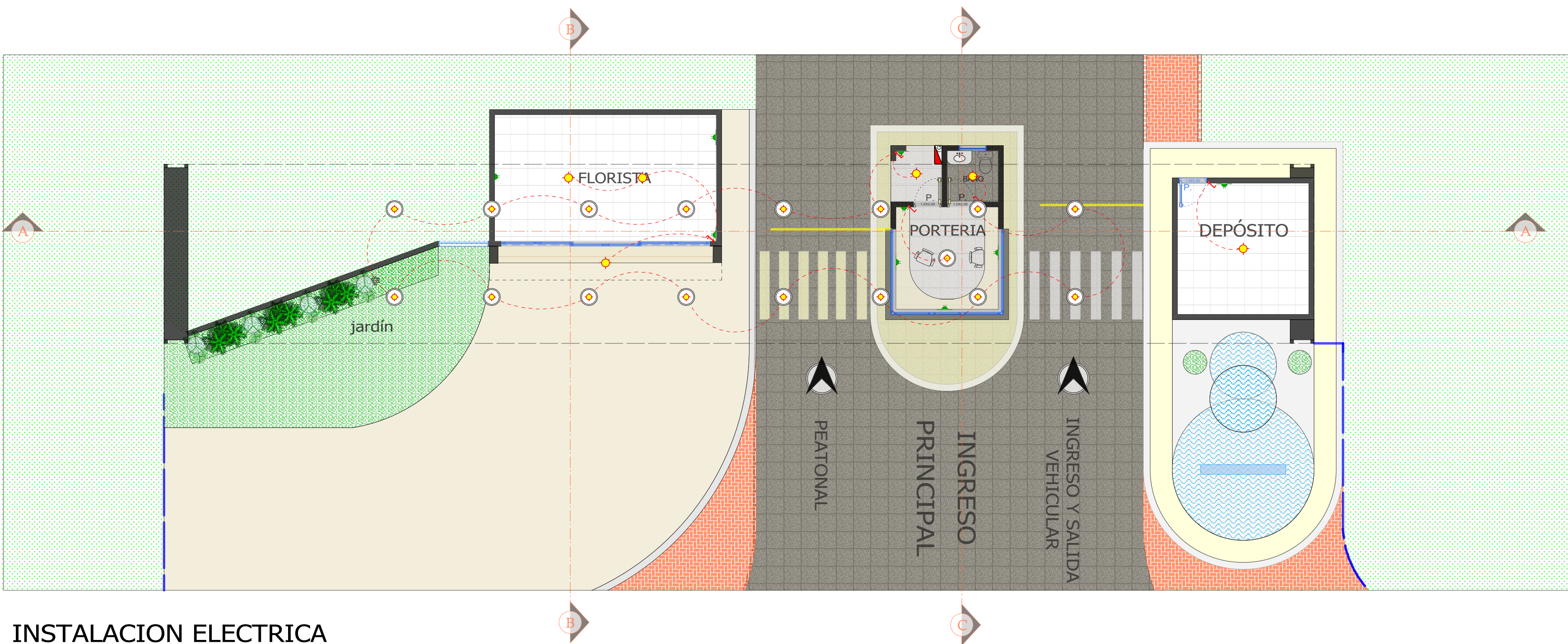
INSTALACION ELECTRICA ESC 1:100
