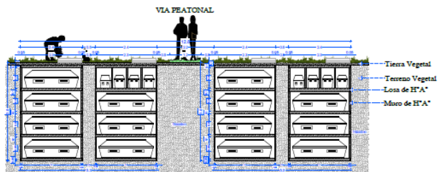
CORTE B-B ESC. 1:50
