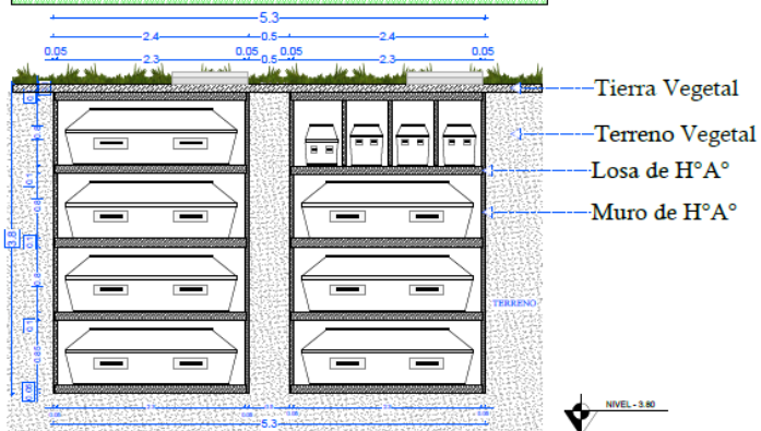
CORTE B-B ESC. 1:25
