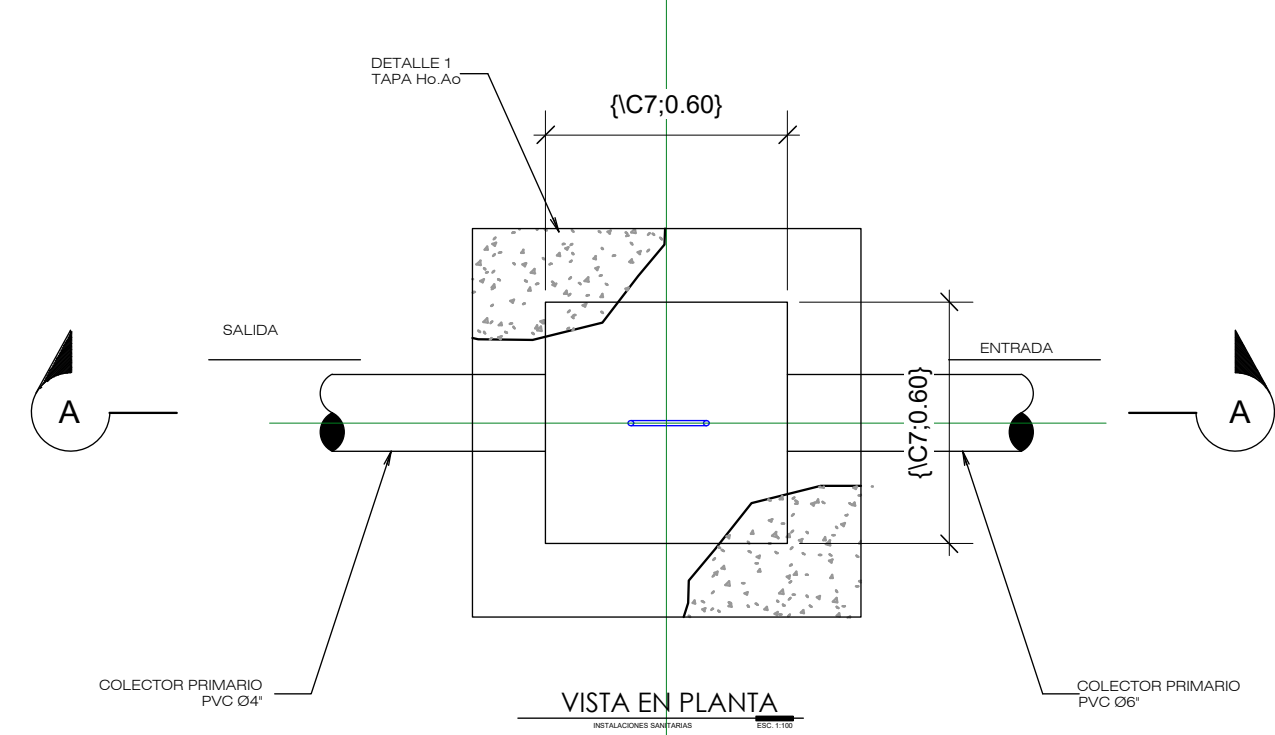
DETALLE CAMARAS DE INSPECCION EXTERIORES ESC. 1:20
