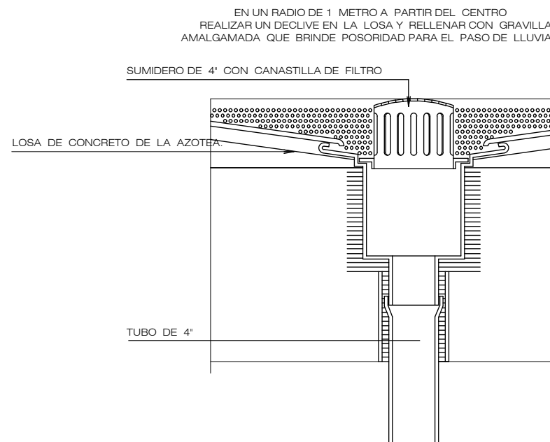
DETALLE - SUMIDERO AZOTEA DETALLE - SUMIDERO AZOTEA
